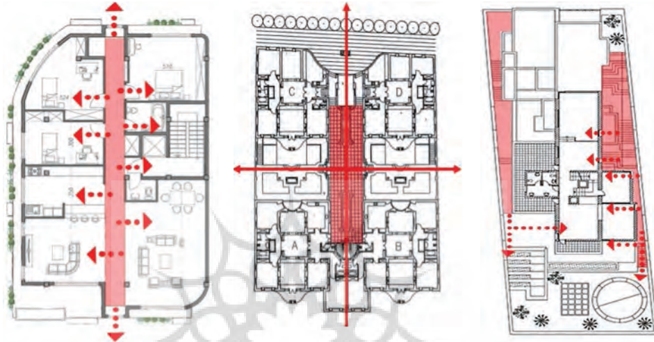
شکل ۱۵. الف) خانه کوهر، پیوند فضاهای باز و بسته و ایجاد تنوع دسترسی از درون به بیرون و بالعکس، منبع: علیزاده، ۱۳۹۶ / ب) مجتمع جلفا، ایجاد ارتباط میان واحدها و حیاطها، قرینه‌سازی فضاها و ایجاد نمودی انتزاعی از کوچه‌های بن‌بست محلات مسکونی با استفاده از انتظام محوری، منبع: www.tajeerarch.com / ج) مجتمع سایه‌ها، تفکیک حریم خصوصی و عمومی با انتظام محوری، کیفیتی دهی به محور حرکتی و برجسته کردن نقش آن با ایجاد ریزفضاهای بسته و باز در طرفین، تنوع در مصالح و رنگ، منتهی شدن به نور و ...، منبع: www.aoapedia.ir
