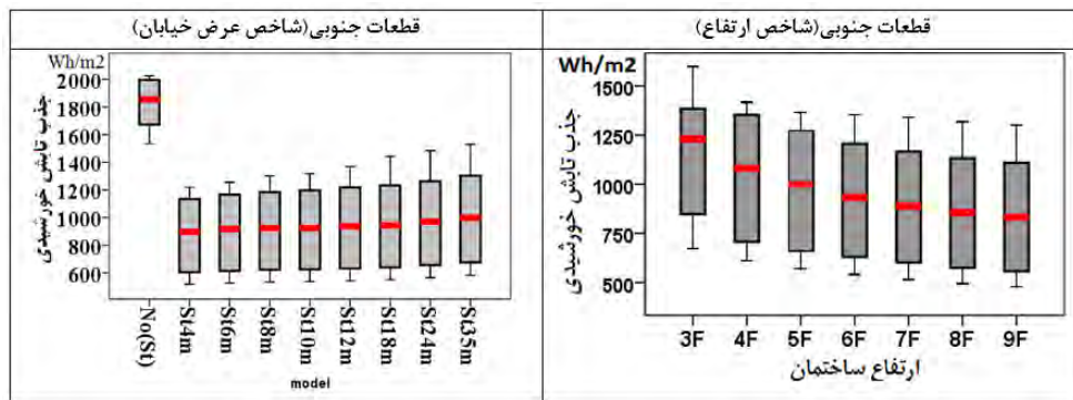
شکل ۱۲. دامنه تغییرات جذب تابش خورشیدی ماهانه شاخص ارتفاع (راست) و شاخص عرض خیابان (چپ) برای قطعات جنوبی. Figure 12. Range of changes in monthly solar radiation absorption height index (right) and street width index (left) for south-ern parts.
