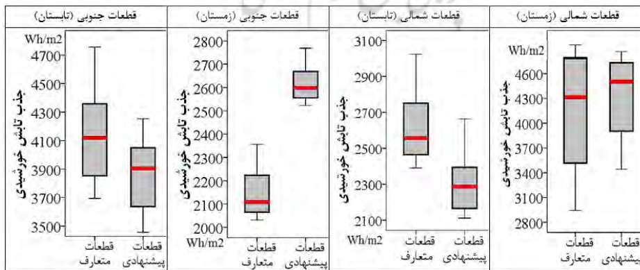
شکل ۱۵. دامنه تغییرات میزان جذب تابش خورشیدی قطعات شمالی و جنوبی الگوی پیشنهادی و متعارف پژوهش در تابستان و زمستان. Figure 15. Range of changes in the amount of solar radiation absorption in the northern and southern parts of the proposed and conventional research model in summer and winter.
