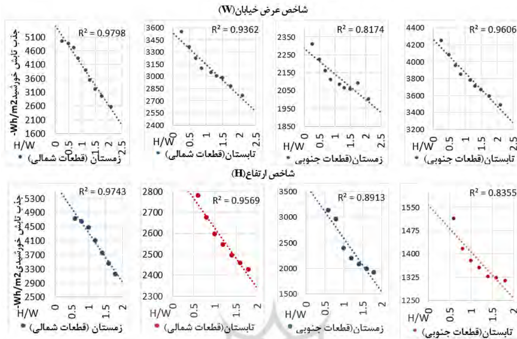
شکل ۱۴. نمودار خطی میزان جذب تابش در تابستان و زمستان برای قطعات جنوبی و شمالی برای شاخص عرض خیابان (ردیف اول) و شاخص ارتفاع (ردیف دوم) مدل پایه پژوهش (ساختمان ۶ طبقه)
