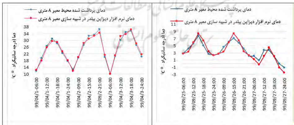
شکل ۱۸. اعتبار سنجی نرم افزار بر اساس دمای برداشت شده و نتایج خروجی شبیه سازی نرم افزار دیژاین بیلدر در معبر ۸ متری - سمت راست آخر آذرماه - سمت چپ اوایل تیرماه.
