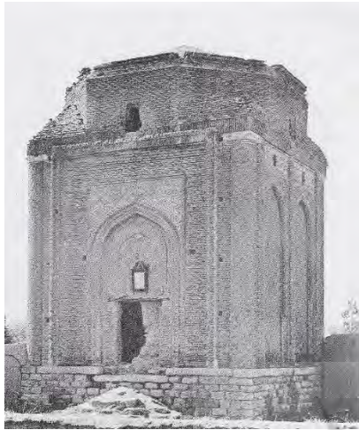
تصویر شماره ۲۱: نمای شمالی گنبد سرخ مراغه (پوپ و آکرمن، ۱۳۸۷ جلد ۸: ۳۴۱)
