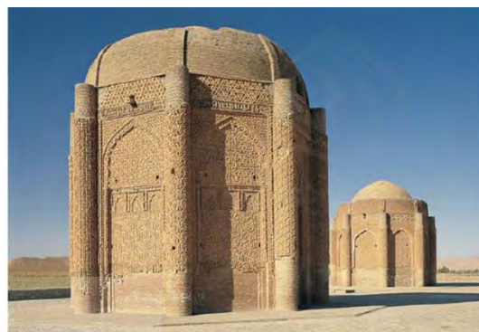
تصویر شماره ۸: نمای برج‌های خرقان آرامگاه نخست، برج غربی و دیگری برج شرقی (افشار، ۱۳۹۷: ۱۴۳)
