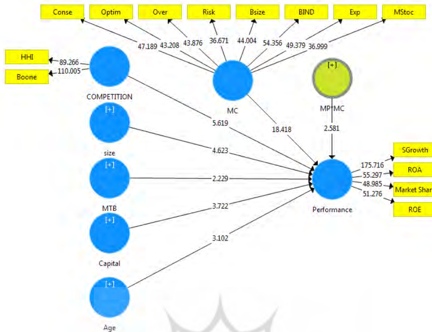
شکل (۲). مقادیر آماره t مدل پژوهش
