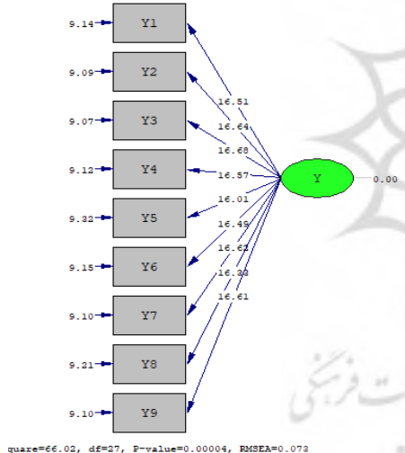
نمودار ۳. اعداد معنی‌داری تحلیل عاملی تأییدی مرتبه اول متغیر عملکرد صادراتی
