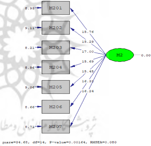
نمودار ۴. اعداد معنی‌داری تحلیل عاملی تأییدی مرتبه اول متغیر نوآوری فنی (توسعه)
