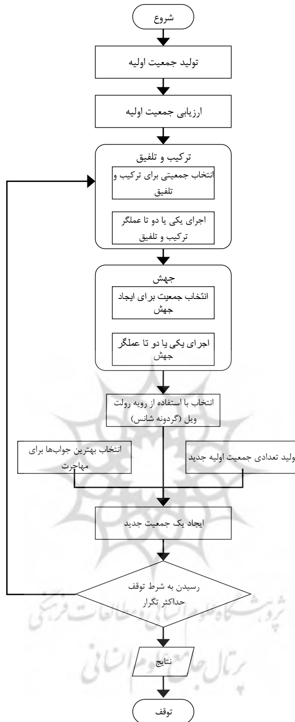
شکل ۱- فلوجارت الگوریتم ژنتیک پیشنهادی
