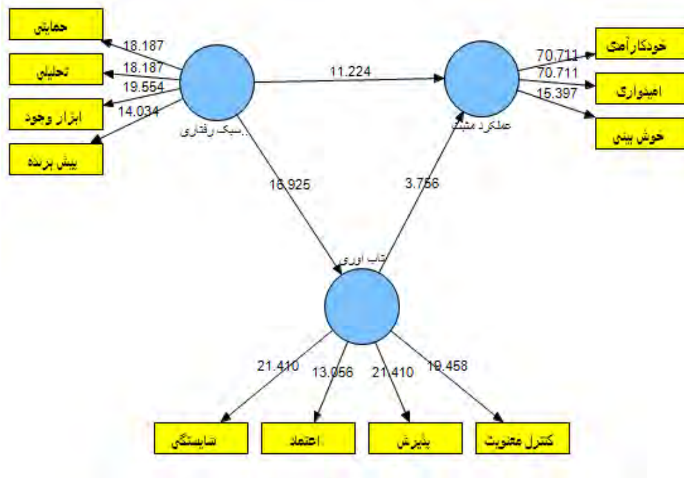
نمودار 2. نمودار آماره تی در حالت معناداری به روش معادلات ساختاری
