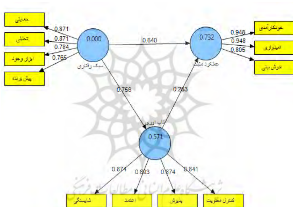
نمودار 1. ضرایب مسیر بین متغیرهای پژوهش به روش معادلات ساختاری
