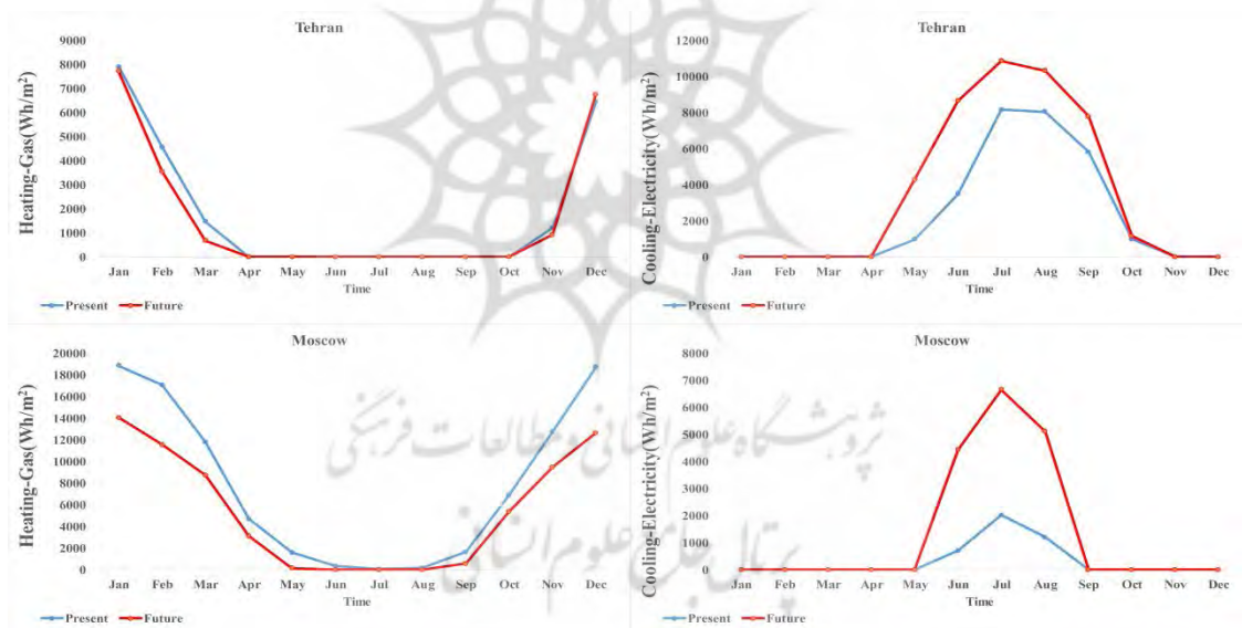
شکل ۹: مقایسه نیاز به انرژی سرمایشی (الکتریسته) و گرمایشی (گاز) برای تهران و مسکو در بستر تغییرات زمانی
