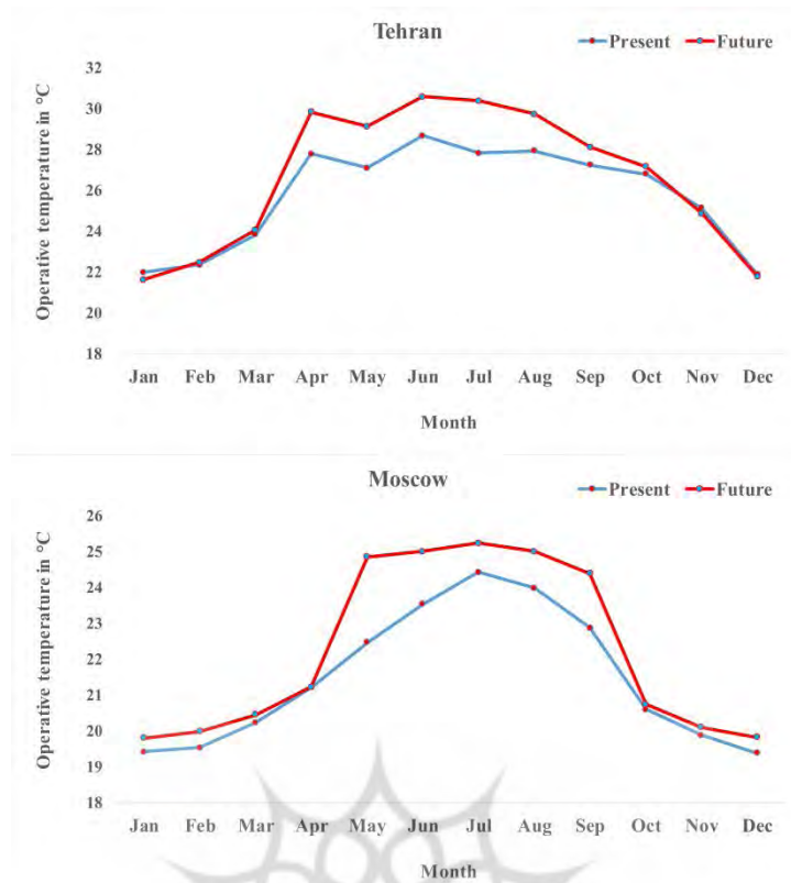
شکل ۷: مقایسه میانگین دمای موثر (OT) برای دوره ی حال و آینده تهران و مسکو
