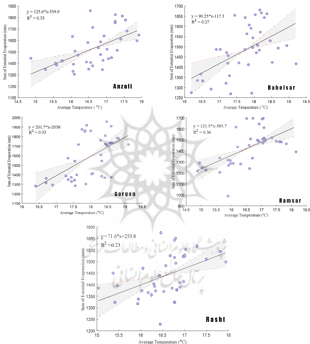
شکل ۵: ارتباط میانگین دما و تبخیر در منطقه مورد مطالعه
