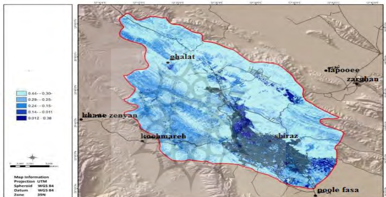
نقشه ۲: نقشه CN حوضه مورد مطالعه
