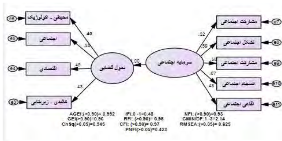
شکل ۳. ساختار تحلیل برازش کلیت اندازه‌گیری متغیرهای وابسته و مستقل پژوهش مأخذ: یافته‌های پژوهش، ۱۳۹۹
