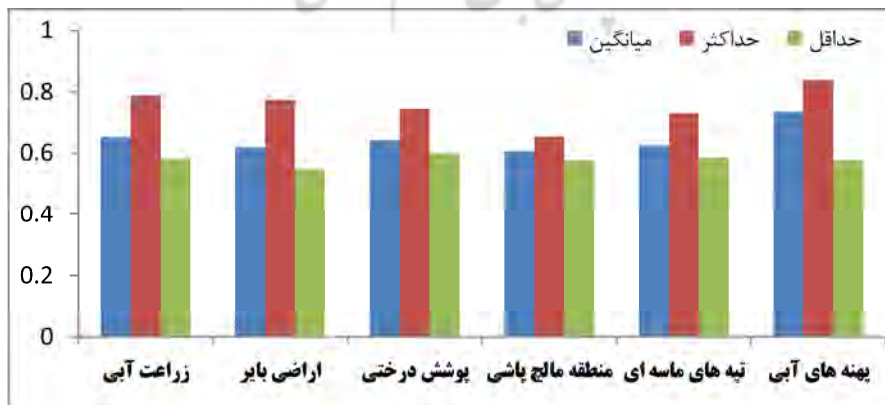
شکل ۲۱. آماره‌های شاخص رطوبت در سال ۲۰۰۱
