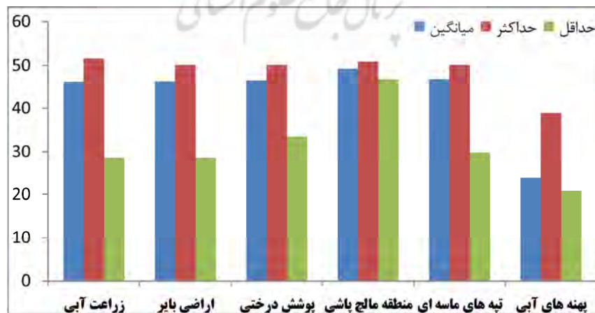
شکل ۱۵. آماره های دمای سطح زمین در سال ۲۰۰۱
