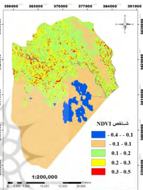
شکل ۶. نقشه شاخص پوشش گیاهی در سال ۲۰۰۱
