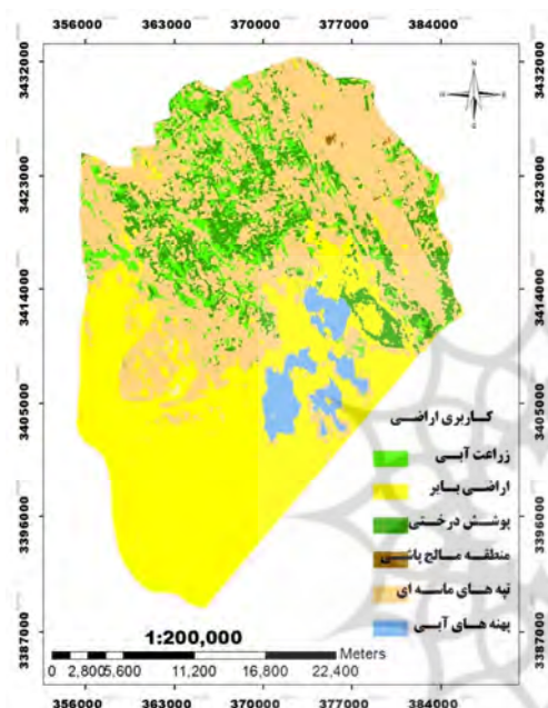
شکل ۳. نقشه کاربری اراضی در سال ۲۰۰۱
