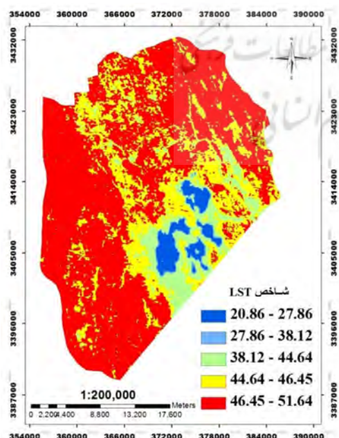
شکل ۱۲. نقشه دمای سطح زمین، سال ۲۰۰۱
