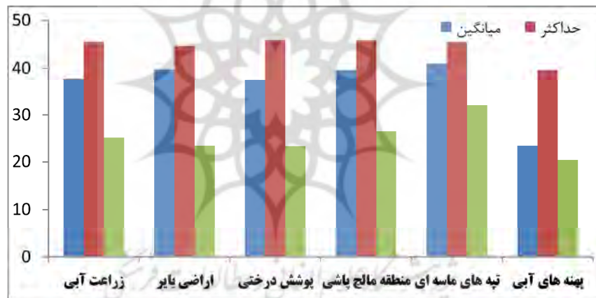
شکل ۱۴. آماره های دمای سطح زمین در سال ۱۹۸۷
