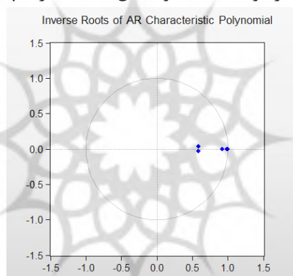
نمودار (۴): شرط پایداری مدل VAR
