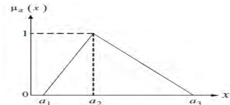
شکل شماره ۱: اعداد فازی مثلثی a
