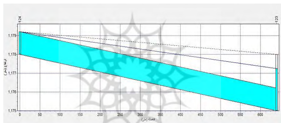
شکل ۷: پروفیل طولی ظرفیت کانال ۱۷ شهریور در دوره بازگشت ۲۰ سال در سرشاخه مجاهدین در وضعیت فعلی
