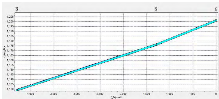
شکل ۶: پروفیل طولی ظرفیت کانال ۱۷ شهریور در دوره بازگشت ۲۰ سال در وضعیت فعلی
