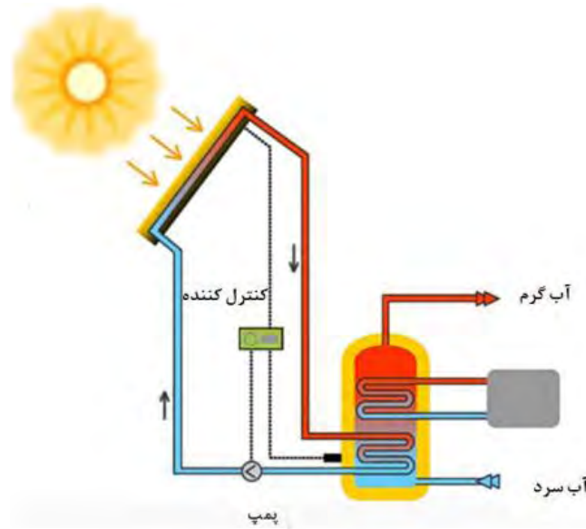
شکل ۱. شماتیکی از سیستم استفاده از گرمایش خورشید
