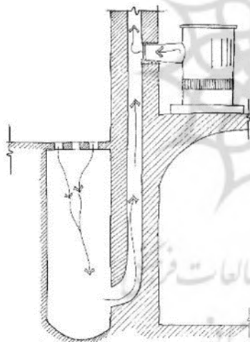
شکل ۵. استفاده از بخاری‌های قدیمی برای بالا بردن قدرت مکش ناکش؛ در تابستان از بادگیر بدین منظور استفاده می‌شده است و بادگیر به صورت مکشی رطوبت را به داخل کشیده و هوای دلپذیری را ایجاد می‌کرده است. (Author, 2022)
