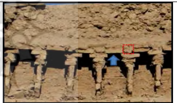
شکل ۱۱. اجرای پوشش پتکین (محلۀ زرتشتیان یزد) به همراه مدل سه‌بعدی
