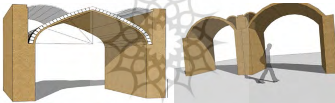
شکل ۳۷. سه‌بعدی از محل مناسب قرارگیری کنو روی شکن‌گاه و سه‌بعدی محل نامناسب قرارگیری کنو روی ایوارگاه منبع: نگارندگان
