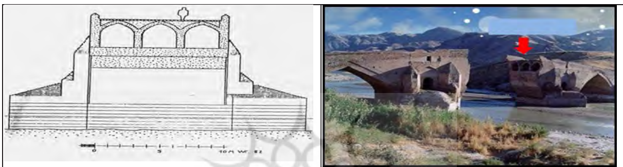
شکل ۴۲. به‌ترتیب کنوی پنهان عمود بر قوس اصلی (پل دختر میانه) و مقطع کنوی پنهان عمود بر قوس اصلی منبع: (Tehrani, 2008)
