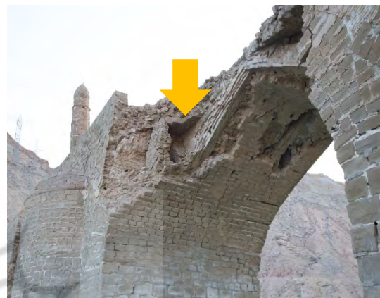
شکل ۳۳. کنو عمود بر طاق اصلی (پل مشیر بوشهر) منبع: نگارندگان
