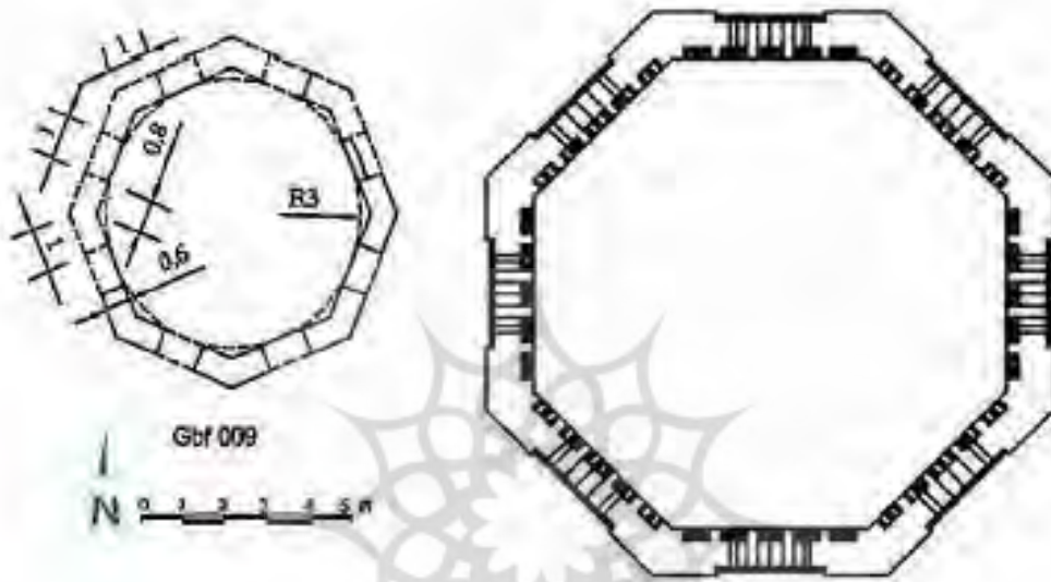
شکل ۱۶. پلان آرامگاه نسک طرح از منصور نجفی
