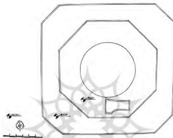
شکل ۴. پلان اصلی گورخانه منبع: آرشیو میراث فرهنگی جیرفت
