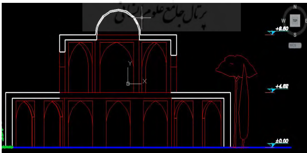
شکل ۱۰. برش عمودی شمالی گورخانه (طراح: فرزاد مجازی، ۱۳۹۶)
