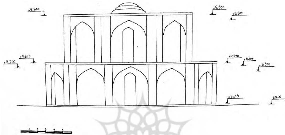
شکل ۶. برش عمودی شرقی گورخانه منبع: آرشيو ميراث فرهنگي جبرفت
