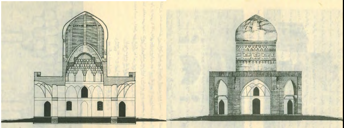
شکل ۲۳. برش عمودی و نمای مقبره ملاحسن کاشی
