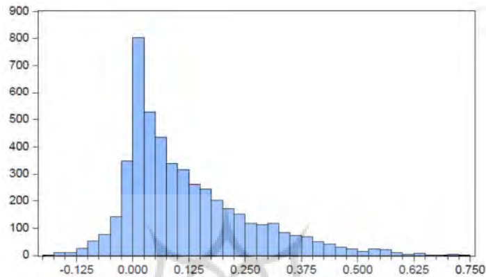
نمودار ۳. هیستوگرام x
