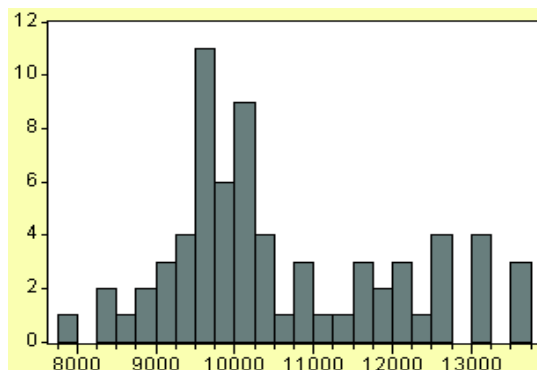
شکل ۴- تابع چگالی تخمینی (شکل بالا) و نمودار هیستوگرام (سمت پایین) شاخص بورس اوراق بهادار تهران در فاصله زمانی ۱۳۸۲-۱۳۸۷
