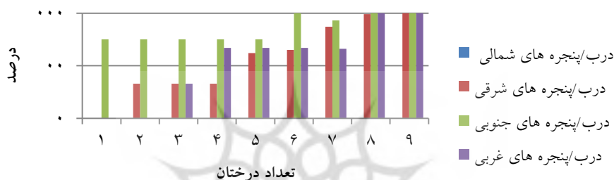
شکل ۸- درصد سایه ایجاد شده بر درب/پنجره‌های شمالی، شرقی، جنوبی و غربی
