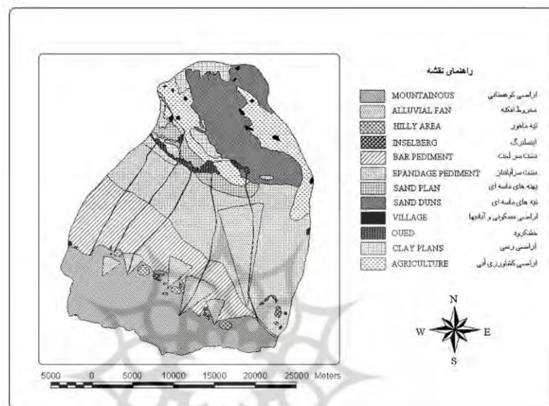
شکل ۲. نقشه ژئومرفولوژی منطقه خضراآباد
