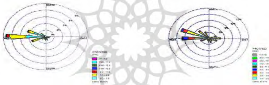
شکل 5- گل‌غبار سالانه ایستگاه همدیدی
