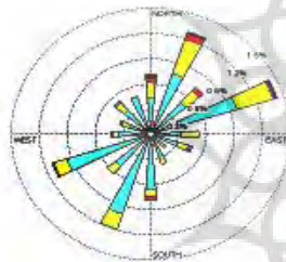
شکل 19- گل غبار اردیبهشت ماه فسا طی دوره آماری 2008-1992
