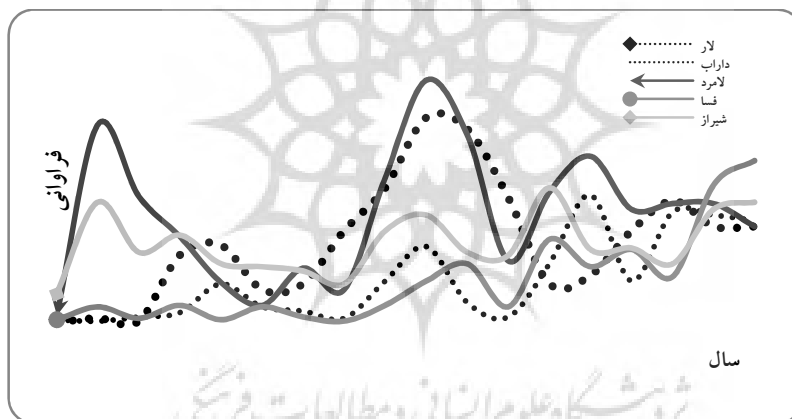
شکل 2- فراوانی سالانه روزهای همراه با گرد و خاک در مناطق جنوب و مرکز استان فارس طی دوره آماری 2008-1992
