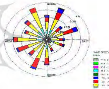
شکل 20- گلباد مرداد ماه فسا طی دوره آماری 2008-1992
