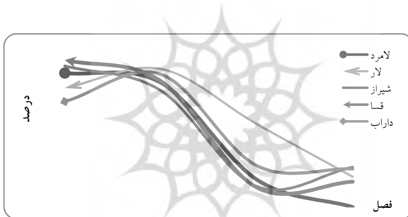
شکل 3- فراوانی فصلی وقوع روزهای همراه با پدیده گرد و غبار در ایستگاه‌های جنوب و مرکز استان فارس طی دوره آماری 1992-2008
