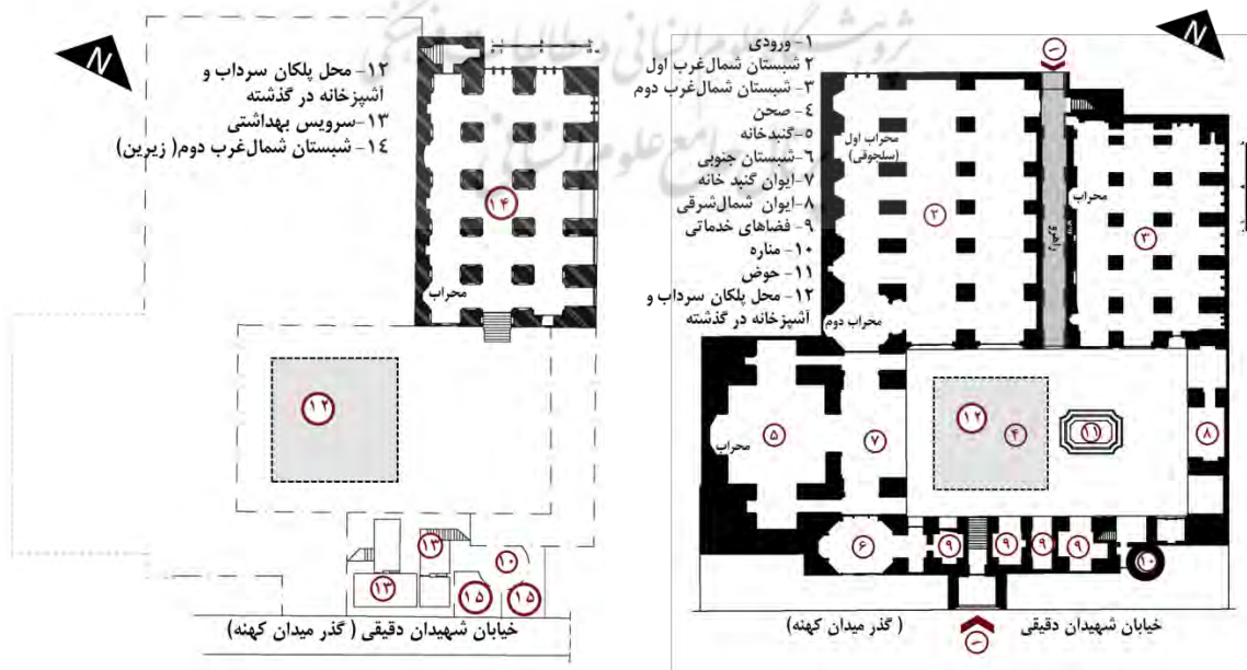
شکل ۴. سمت راست: پلان طبقه همکف. سمت چپ: پلان طبقه زیرزمین (اصلاحات نگارندگان بر روی نقشه‌های موجود در اداره میراث فرهنگی شهرستان کاشان)
