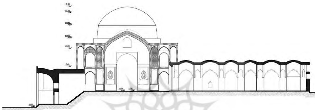
شکل ۵. بالا: برش افقی از حیاط (اداره میراث فرهنگی کاشان)، پایین: برش عمودی از حیاط (اصلاحات نگارندگان بر روی نقشه میراث فرهنگی کاشان)
