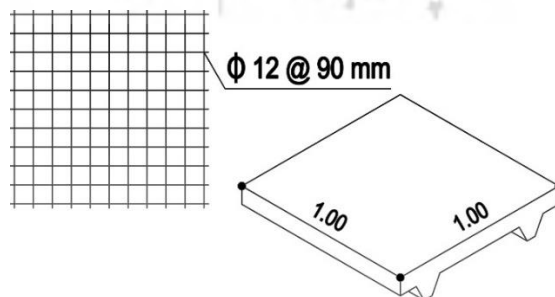
تصویر ۶- جزئیات صفحات بتنی (کف بتنی)
