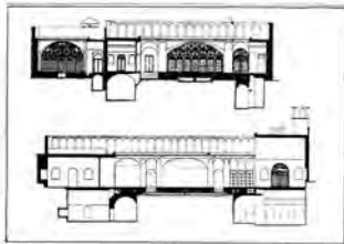
۶- مقاطع خانه رسولیان
