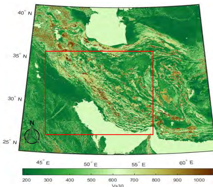
شکل (۱): مستطیل مورد استفاده جهت استخراج داده‌های مربوط به میانگین سرعت موج برشی در سی متر اول زیر سطح ( V_{s30} )
