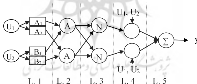
شکل ۱: معماری شش‌گانه شبکه استنتاج عصبی فازی تطبیق پذیر (ANFIS) (Kimiaefar et Al 2018)
