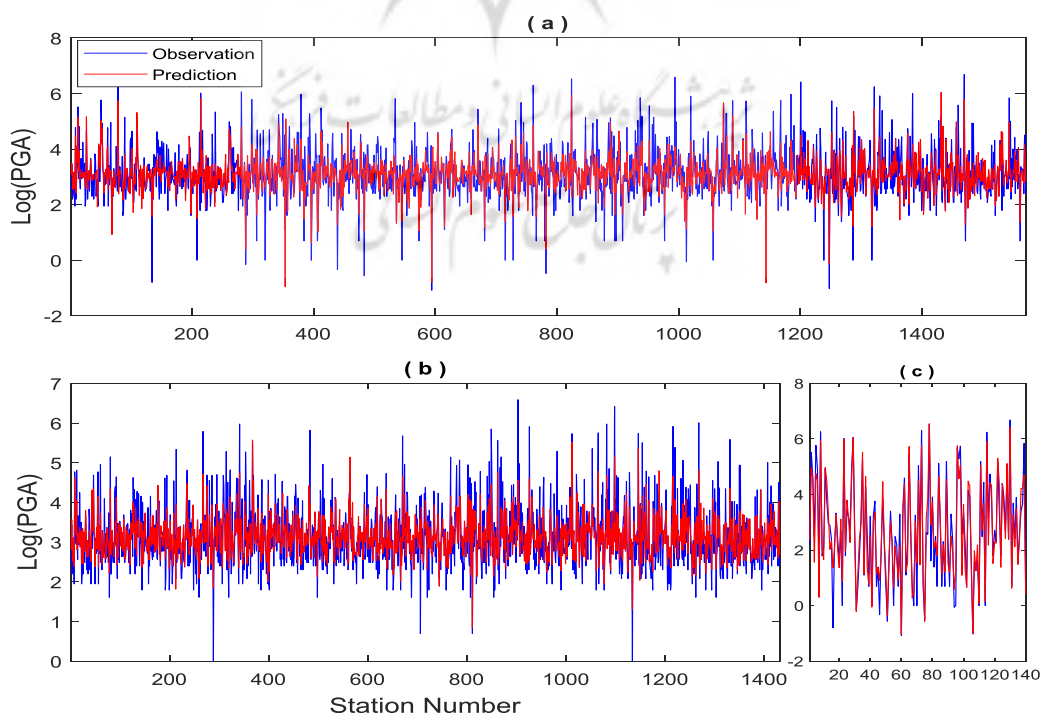
شکل (۵): مقادیر هدف و خروجی شبکه انفیس برای داده‌های مورد استفاده بدون تفکیک (a)، گروه داده‌های متجانس (b) و نامتجانس (c). نسبت به شکل ۳، در اینجا تاکید فرآیند آموزش با داشتن بالاترین عملکرد برای تعمیم داده‌ها بر روی داده‌های تست بوده است.
