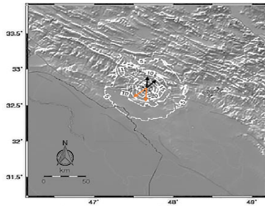
شکل (۱۰): نقشه توزیع بیشینه شتاب زمین گزارش شده توسط پژوهشگاه بین‌المللی زلزله‌شناسی و مهندسی زلزله برای زلزله مورموری (۲۷ مرداد ۱۳۹۳). کنتورهای رسم شده بر اساس درصد شتاب نقل می‌باشند. جهت‌نماهای سیاه و نارنجی هر کدام به ترتیب نمایش‌دهنده فاصله بین رومرکز تا خط کنتور هم شدت ۱۵ درصد شتاب نقل می‌باشند که در جهات مختلف با رنگ متمایز رسم شده‌اند تا امکان مقایسه جهت‌گیری کلی توزیع PGA میسر گردد. توجه شود که جهت‌نماهای نارنجی طول بزرگتری دارند.
