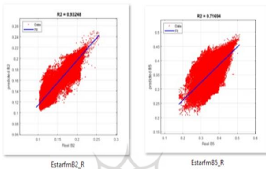
خروجی ESTARFM
