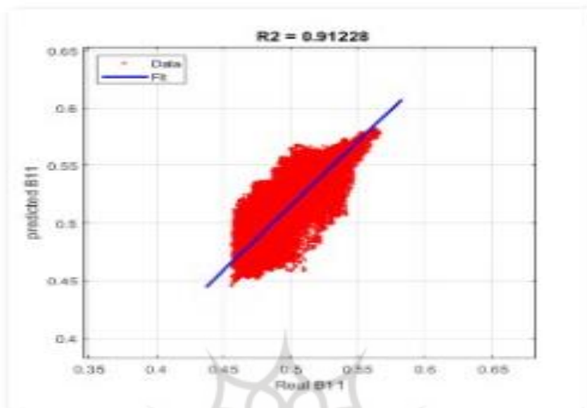
خروجی SADFAT
