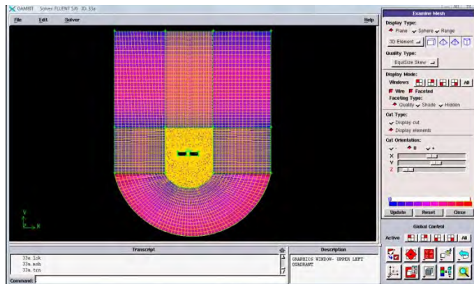
شکل ۶. مدل‌سازی در نرم‌افزار گمبیت ۲/۲ منبع: نگارندگان
