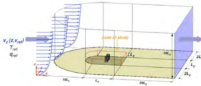
شکل ۵. گام اول، تعریف حوزه تحت تأثیر باد بر اساس استاندارد AIJ منبع: نگارندگان
