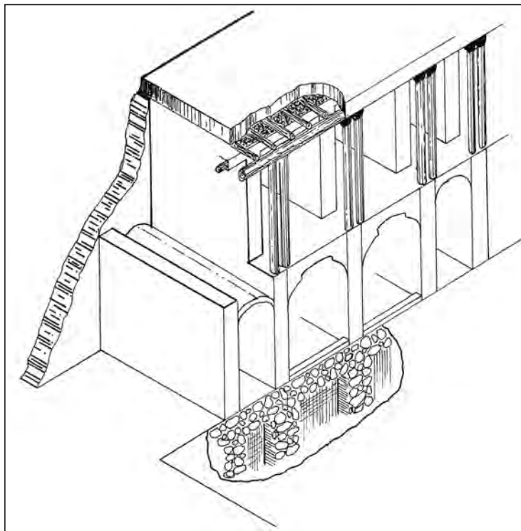
شکل ۸. نمایش ساختار مرکب سیستم سازه‌ای، سرای حاج محمدقلی بازار تبریز
