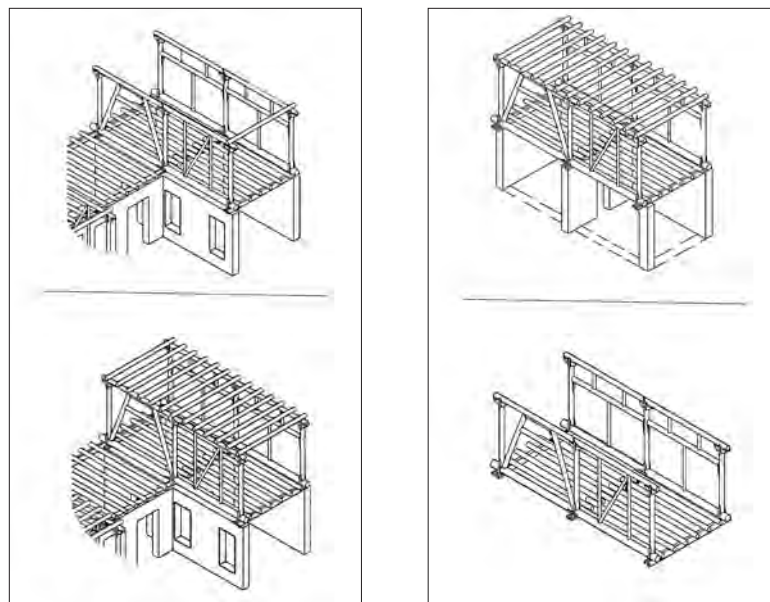
شکل ۹ و ۱۰: تحلیل شماتیک موقعیت عضوهای قطری در سیستم کلاف‌بندی چوبی خانه‌های قاچاری
