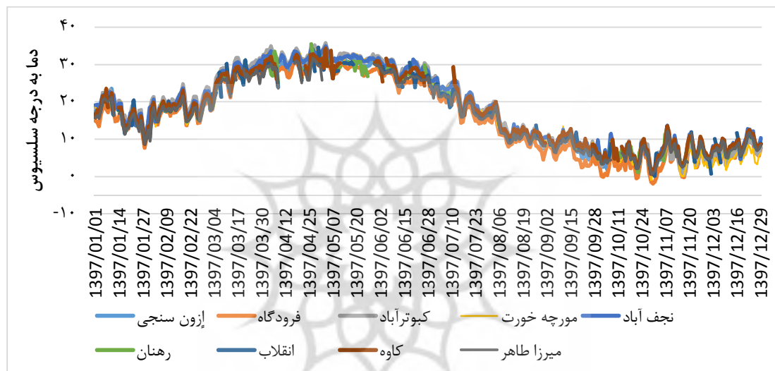
شکل ۳: انطباق خط روند تغییرات روزانه دما در چهار ایستگاه هوا-آلوده‌سنجی مرکز پایش
