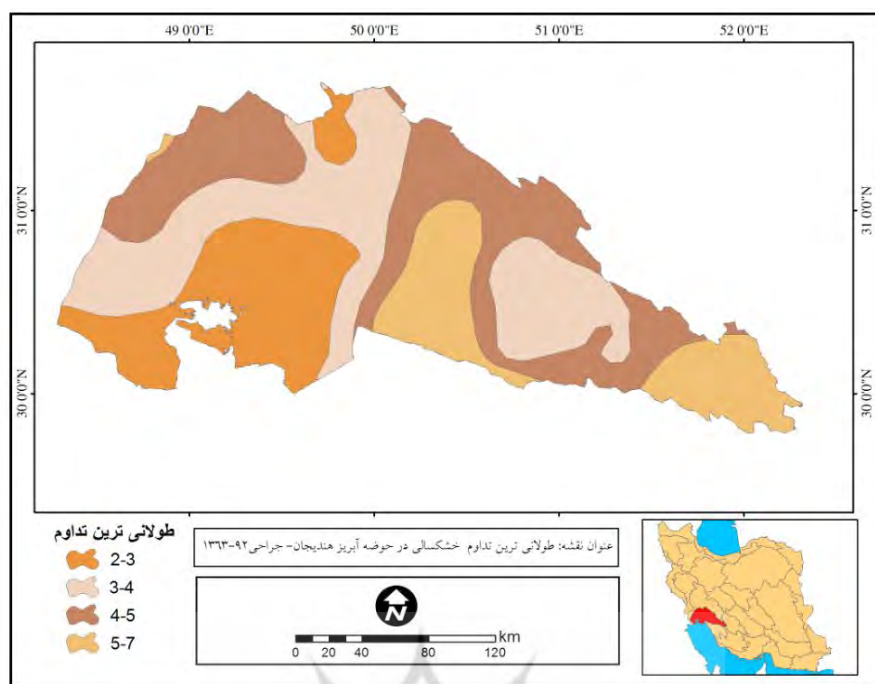
شکل ۳: پهنه‌بندی طولانی‌ترین تداوم رخداد خشکسالی در حوضه آبریز هنديجان-جراحی
