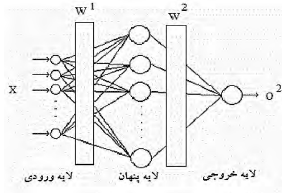
شکل ۶: ساختار معماری شبکه عصبی چند لایه (MLP) (منبع: یافته‌های پژوهش، ۱۳۹۶)
