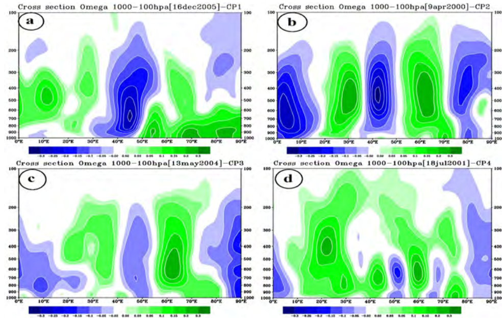
شکل ۱: وضعیت سرعت قائم (شاخص امگا) در هر الگو. شکل a مربوط به الگوی نخست: روز نماینده ۱۶ دسامبر ۲۰۰۵ - شکل b مربوط به الگوی دوم: روز نماینده ۹ آوریل ۲۰۰۰ - شکل c مربوط به الگوی سوم: روز نماینده ۱۳ می ۲۰۰۴ - شکل d مربوط به الگوی چهارم: روز نماینده ۱۸ جولای ۲۰۰۱.
