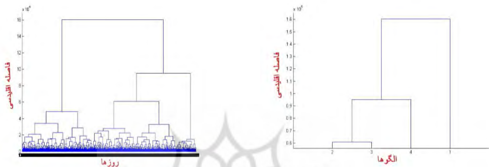
شکل ۴: دارنمای کلی الگوهای گردشی در زمان رخداد بارش روزانه و فراگیر
