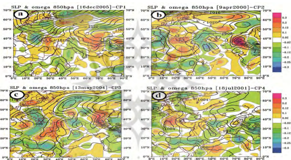
شکل ۷: وضعیت فشار تراز دریا و سرعت قائم (امگا) در الگوهای گردشی. شکل a مربوط به الگوی نخست: روز نماینده ۱۶ دسامبر ۲۰۰۵- شکل b مربوط به الگوی دوم: روز نماینده ۹ آوریل ۲۰۰۰- شکل c مربوط به الگوی سوم: روز نماینده ۱۳ می ۲۰۰۴- شکل d مربوط به الگوی چهارم: روز نماینده ۱۸ جولای ۲۰۰۱.
