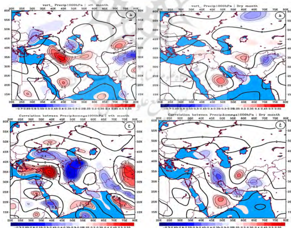
شکل ۷: همبستگی بین بارش و تاوایی تراز ۱۰۰۰ ه.پ در ماه مرطوب (ط) و ماه خشک (ظ) بارش و صعود قائم تراز ۱۰۰۰ ه.پ در ماه مرطوب (ع) و ماه خشک (غ)
