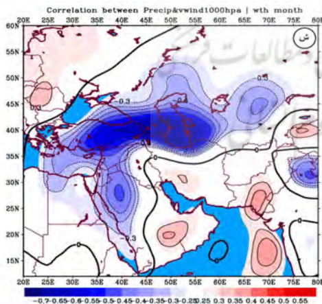
شکل ۶: همبستگی بین بارش و مؤلفه باد نصف‌النهاری تراز ۱۰۰۰ ه.پ در ماه مرطوب (ش) و ماه خشک (ص)
