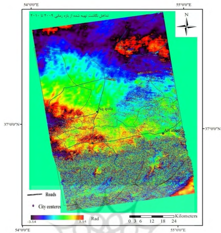
شکل ۳: تداخل نگاشت تهیه شده در بازه زمانی ۲۰۰۹ تا ۲۰۱۰، جایجایی در راستای دید ماهواره
