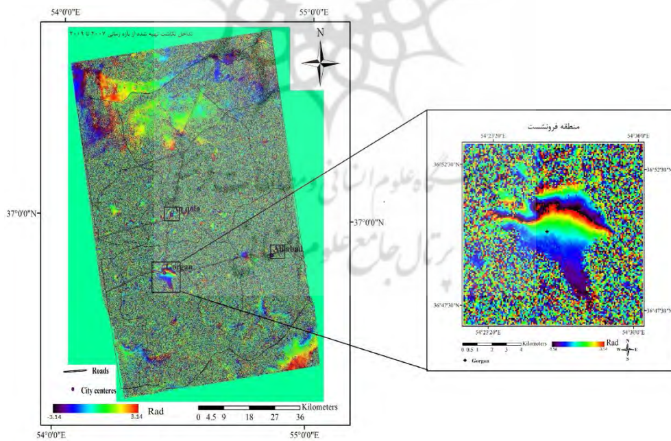
شکل ۴: تداخل نگاشت تهیه شده در بازه زمانی ۲۰۰۷ تا ۲۰۰۹، جایجایی در راستای دید ماهواره
