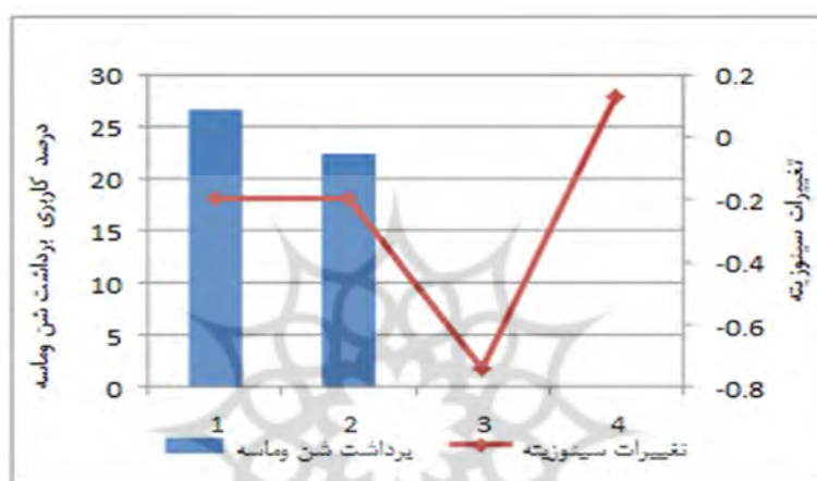
شکل ۹: نمودار ارتباط کاربری برداشت شن و ماسه با تغییرات سینوزیته بازه‌ها
