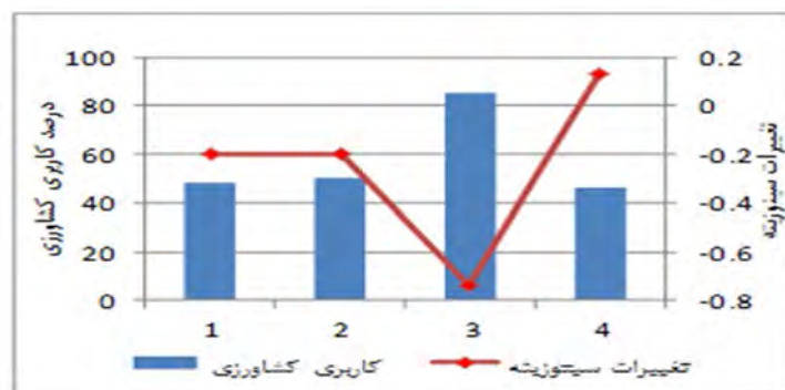
شکل ۷: نمودار ارتباط کاربری کشاورزی با تغییرات سینوزیته بازه‌ها
