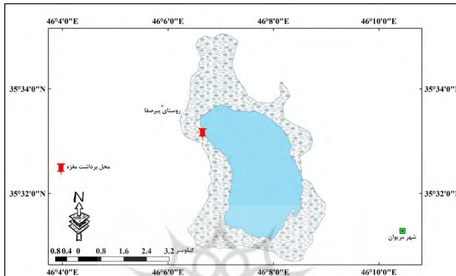
شکل ۱- محل و موقعیت برداشت مغزه‌ی رسوبی
