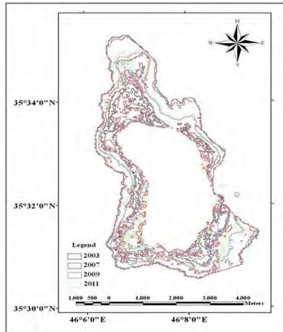
شکل ۸- تغییرات خط ساحلی دریاچه زیروار طی سال‌های ۲۰۰۳ تا ۲۰۱۱ برای بازسازی اکوتومورفولوژی عهد حاضر
