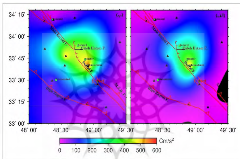
شکل ۴- پهنه‌های هم‌شتاب زمین‌لرزه سیلاخور با استفاده از شتاب‌های ثبت شده در ایستگاه‌های شتاب‌نگاری متعلق به مرکز تحقیقات ساختمان و مسکن (برگرفته از رضایپور، ۱۳۸۸). (الف) برای مولفه قائم (ب) برای مولفه افقی.
