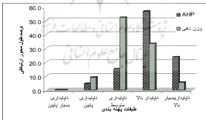
شکل ۷- درصد مسافت ناپایداری طبقات پهنه‌بندی جاده اصلی ساندج- مریوان.
