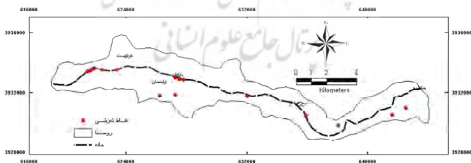
شکل ۲- پراکنش زمین لغزش‌ها جاده اصلی سنندج- مریوان
