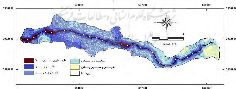
شکل ۵ - پهنه‌بندی خطر زمین لغزش جاده اصلی سنندج - مریوان به روش تحلیل سلسله مراتبی
