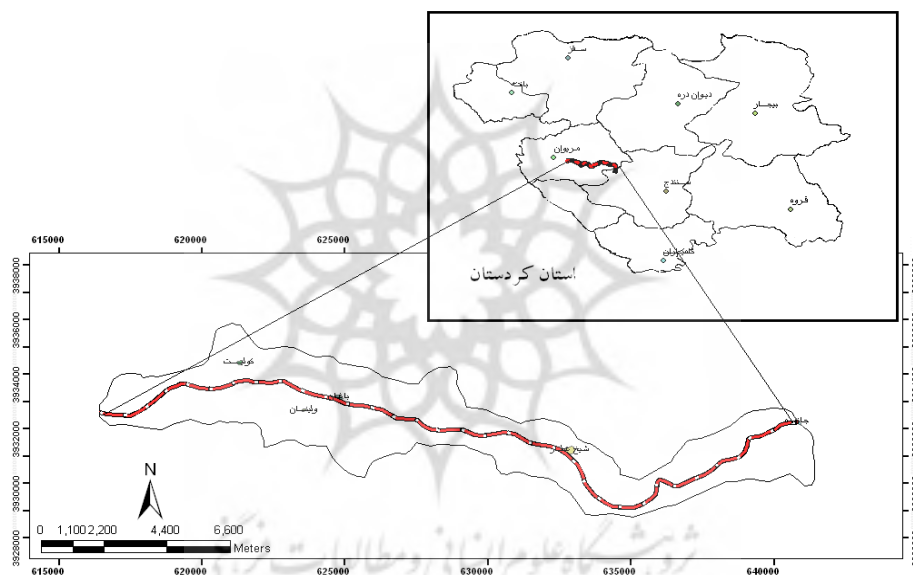
شکل ۱- موقعیت مسیر مورد مطالعه
