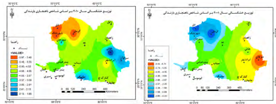
شکل ۲: توزیع خشکسالی بر اساس نمایه RAI طی شدیدترین و فراگیرترین الف: سال ۲۰۰۱، ب: سال ۲۰۱۰
