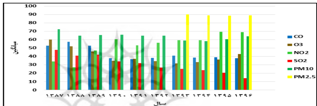
شکل ۲: میانگین سالانه روند تغییرات غلظت آلاینده‌ها در دوره آماری (۱۳۸۶-۱۳۹۶). منبع: نگارنده)
