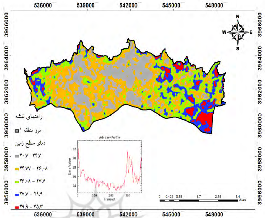
شکل ۶: دمای رویه سطح زمین (LST) و پروفایل دمایی از غرب به شرق منطقه (۱۹ اکتبر ۲۰۱۹) منبع: (نگارنده) شکل ۸ تصویر ماهواره‌ای دمای سطحی زمین را در منطقه یک تهران برای روز ۵ فوریه (۱۶ بهمن) نشان می‌دهد. با وجود اینکه در این تصویر ما در یک ماه زمستانی قرار داریم و تقریباً در اکثر بخش‌ها پوشش درختی فاقد برگ و سبزینه می‌باشد ولی همچنان بخش جنوب شرقی از دمای سطحی بالاتری نسبت به سایر بخش‌های منطقه برخوردار است. دمای سطحی در این بخش به بیش از ۱۵ درجه سانتی‌گراد نیز می‌رسد.
