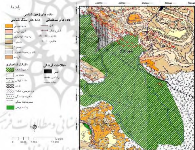
شکل ۱: نقشه ژئومورفولوژی محدوده کلانشهر کرج
