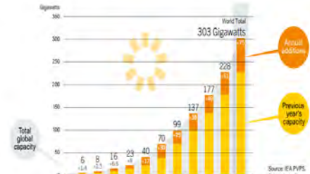
شکل ۱: میزان تجمعی سامانه‌های فتولتائیک در جهان
