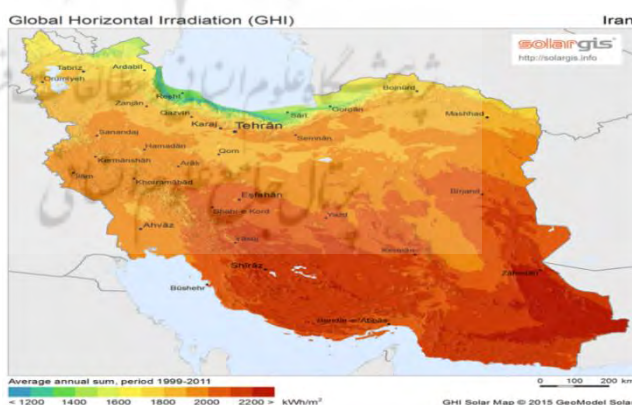
شکل ۳: میزان تابش کل سالانه کشور ایران بر مبنای \text{kWh/m}^2 (منبع: GHI)
