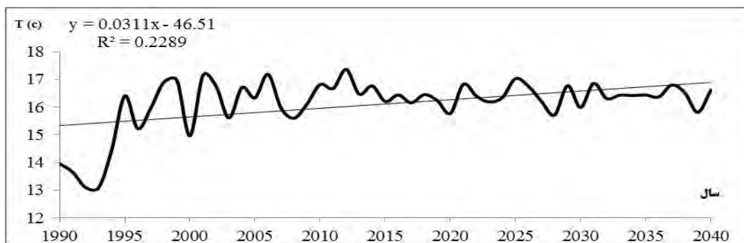
شکل ۴: میانگین دمای بیشینه سالانه ایستگاه اردبیل در دوره پایه (۱۹۹۰-۲۰۱۰) و پیش‌بینی شده (۲۰۱۱-۲۰۴۰)
