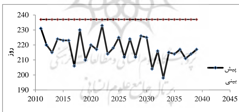
شکل ۷: مقایسه میانگین بلندمدت طول دوره رشد گندم دیم در دوره پایه (۱۹۹۰-۲۰۱۰) با طول دوره رشد گندم دیم در سال‌های آینده (۲۰۱۱-۲۰۳۹) منبع: یافته‌های پژوهش، ۱۳۹۶
