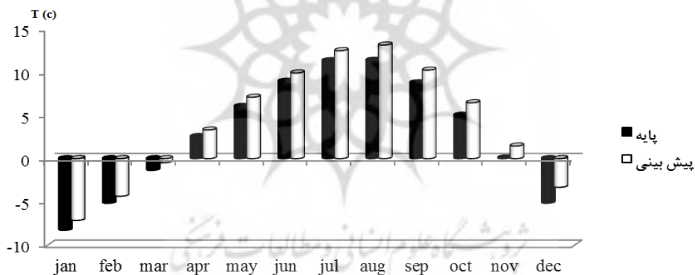
شکل ۳: مقایسه میانگین بلندمدت دمای کمینه ماهانه در دوره پایه (۱۹۹۰-۲۰۱۰) با دوره پیش‌بینی شده (۲۰۱۱-۲۰۴۰)
