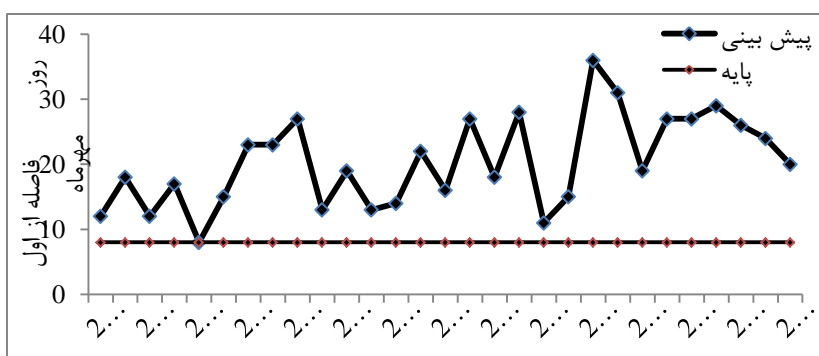
شکل ۶: مقایسه میانگین بلندمدت تاریخ‌های آغاز کشت گندم دیم بر اساس فاصله از مبدأ (اول مهر) در دوره پایه (۱۹۹۰-۲۰۱۰) با تاریخ‌های آغاز کاشت در سال‌های آینده (۲۰۱۱-۲۰۳۹) منبع: یافته‌های پژوهش، ۱۳۹۶
