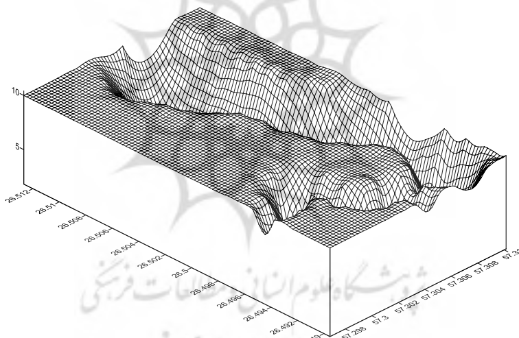
شکل ۱۱: نمایش سه بعدی (3D) مخزن سد زیرزمینی پیشنهادی با استفاده از نرم افزار Surfer v.10.0
