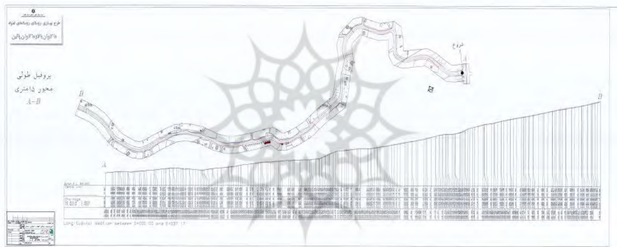
شکل ۳. نیمرخ و بروئیل طولی ماسوله رودخان در امتداد شهر ماکلوان (منبع مهندسین مشاور بزرگ امید)
