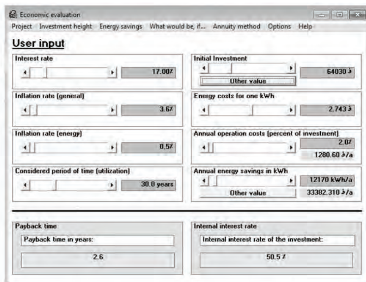
شکل ۱۰. تحلیل اقتصادی با نرم‌افزار OekoRat در راستای استفاده از نوع و نسبت بهینه پنجره در ساختمان با استفاده از متوسط هزینه‌های انرژی جهانی
