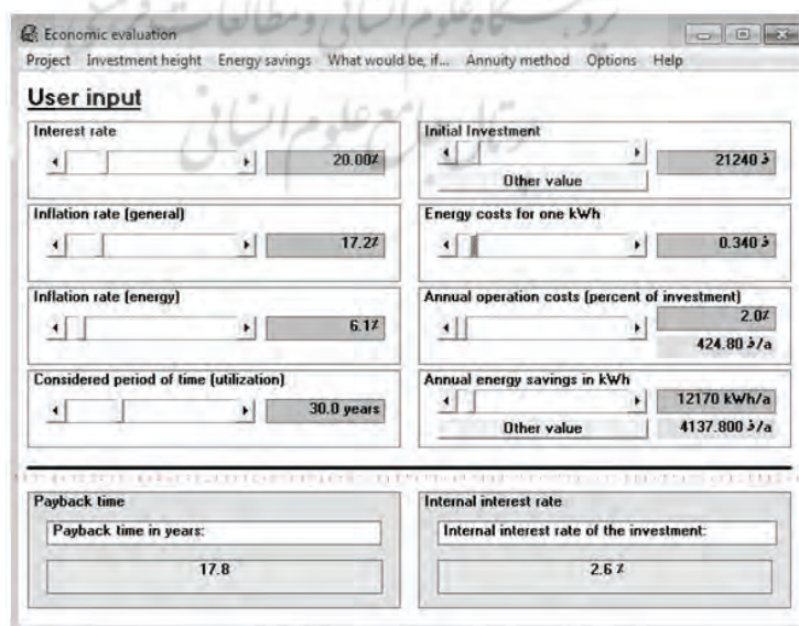
شکل ۹. تحلیل اقتصادی با نرم‌افزار OekoRat در راستای استفاده از نوع و نسبت بهینه پنجره در ساختمان با استفاده از نرخ هزینه‌های انرژی در ایران
