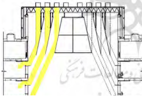
شکل ۹. چیدمان منعکس کننده‌های قابل تنظیم، روی سقف آتریوم شکل ۱۰. نحوه‌ی انتقال نور به فضاهای کناری آتریوم با استفاده از سه نوع منعکس کننده
